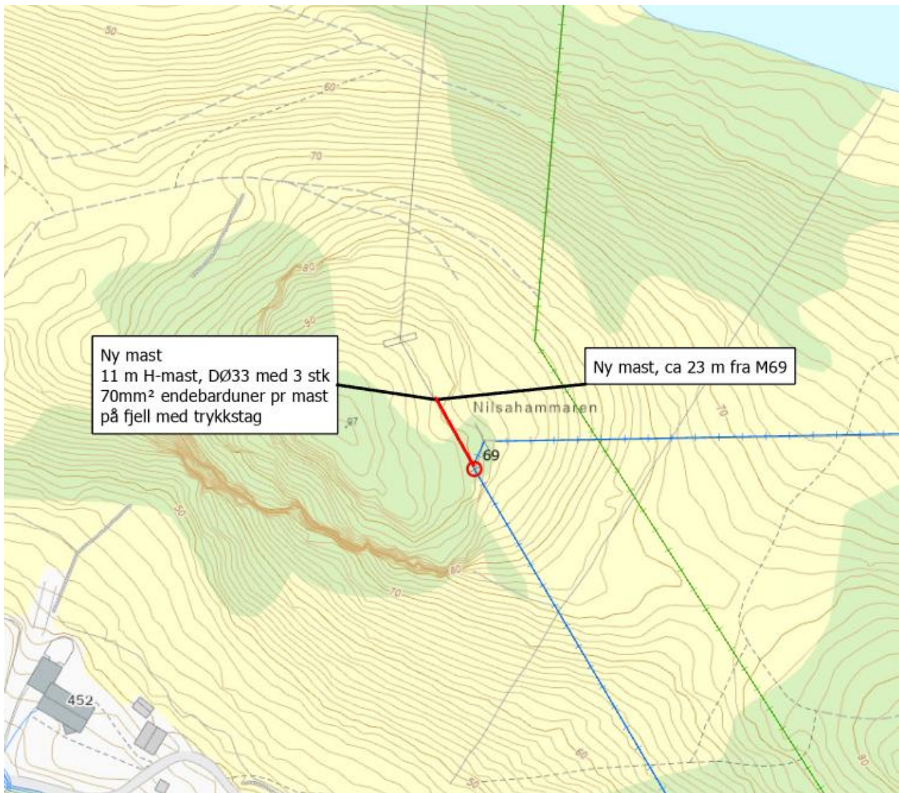
Figur 3 Detaljkart etter riving område mast 69-70, Nilsahammaren
