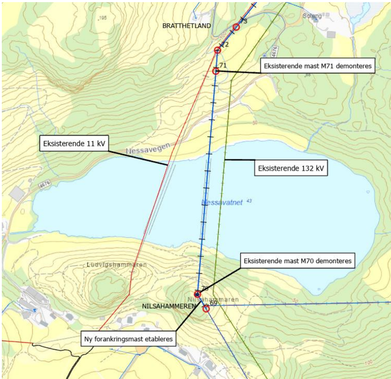
Figur 2 Detaljkart riving område mast 69-73, Nessavatnet
